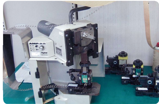
▲ 圧着機
